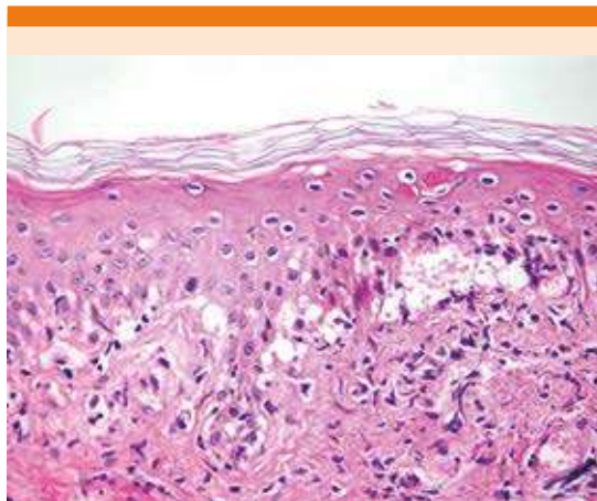
Figura 3. Microscopia de luz teñida con hematoxilina y eosina que muestra ortoqueratosis laminar, aplastamiento de los procesos interpapilares, vacuolización masiva de la membrana basal que llega a formar hendiduras en la dermis superficial y profundo infiltrado inflamatorio linfocitos e histiocitos.
